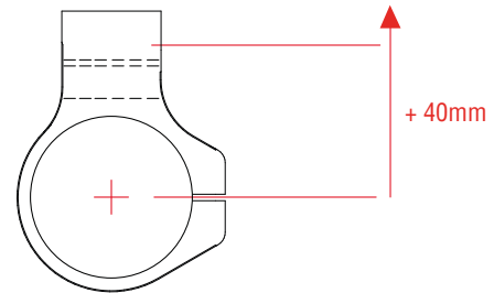
Bracelets de guidons avec décalage +40 mm Lenkerschellen mit Offset +40mm
